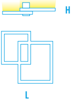
2160/PL60-1 W 66 - Vac 230 Lm 4.800 L 600 x 600 mm H 160 mm
