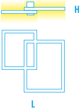
2160/PL80-2 W 168 - Vac 230 Lm 12.000 L 800 x 800 mm H 160 mm
