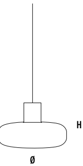
2151/S5 1 x E27 Ø 450 mm H 260 mm L CAVO / CABLE 3.000 mm
