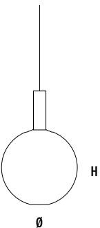
2158/S2 1 x E27 Ø 400 mm H 550 mm L CAVO / CABLE 3.000 mm
