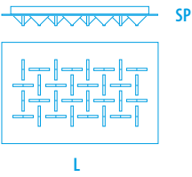
2052/PL 80 W 70 - Vac 230 Lm 5.200 L 500 x 800 mm SP 80 mm
